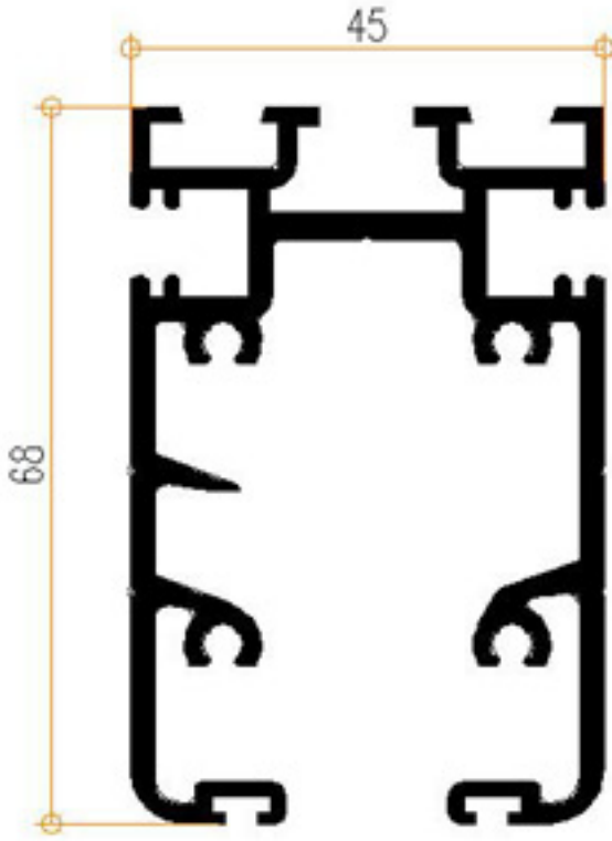
ÜST RAY PROFİLİ 6503
