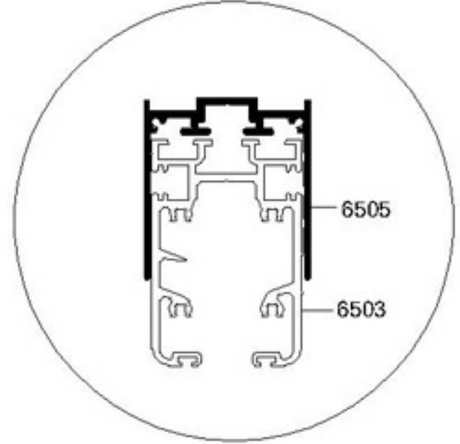
ÜST RAY PROFİLİ 6503
